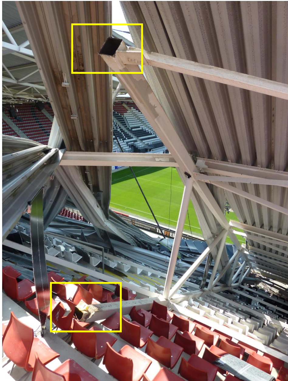
Overzicht bezweken lasverbindingen boven- en onderspant van één van de vier spanten
